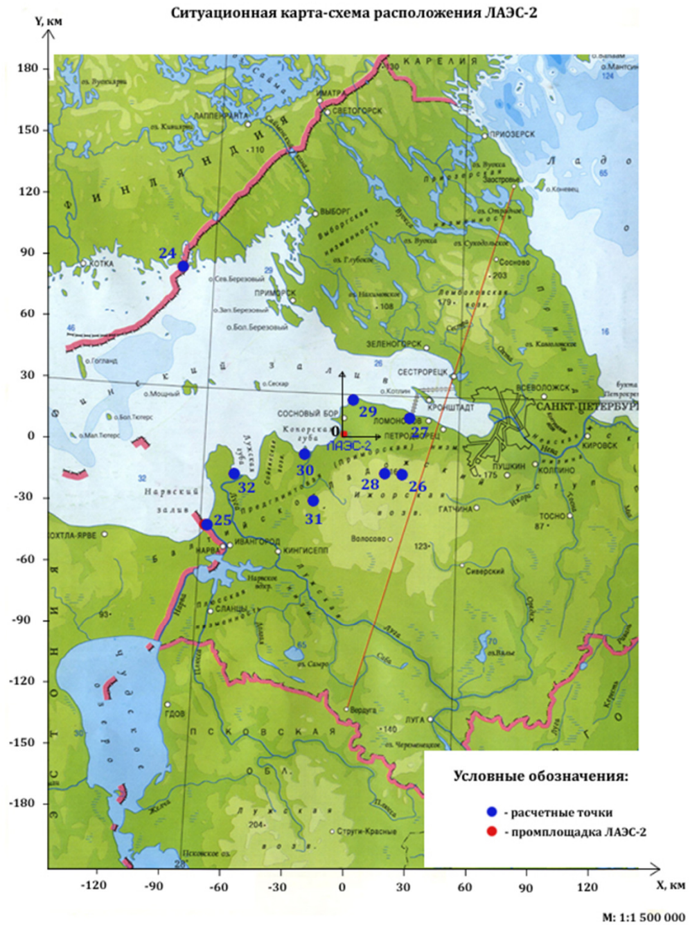
Рисунок 5.4.1.1.1 – Расчетные точки рассеивания в районе расположения Ленинградской АЭС-2 на границах Финляндии и Эстонии, ООПТ (при эксплуатации)
