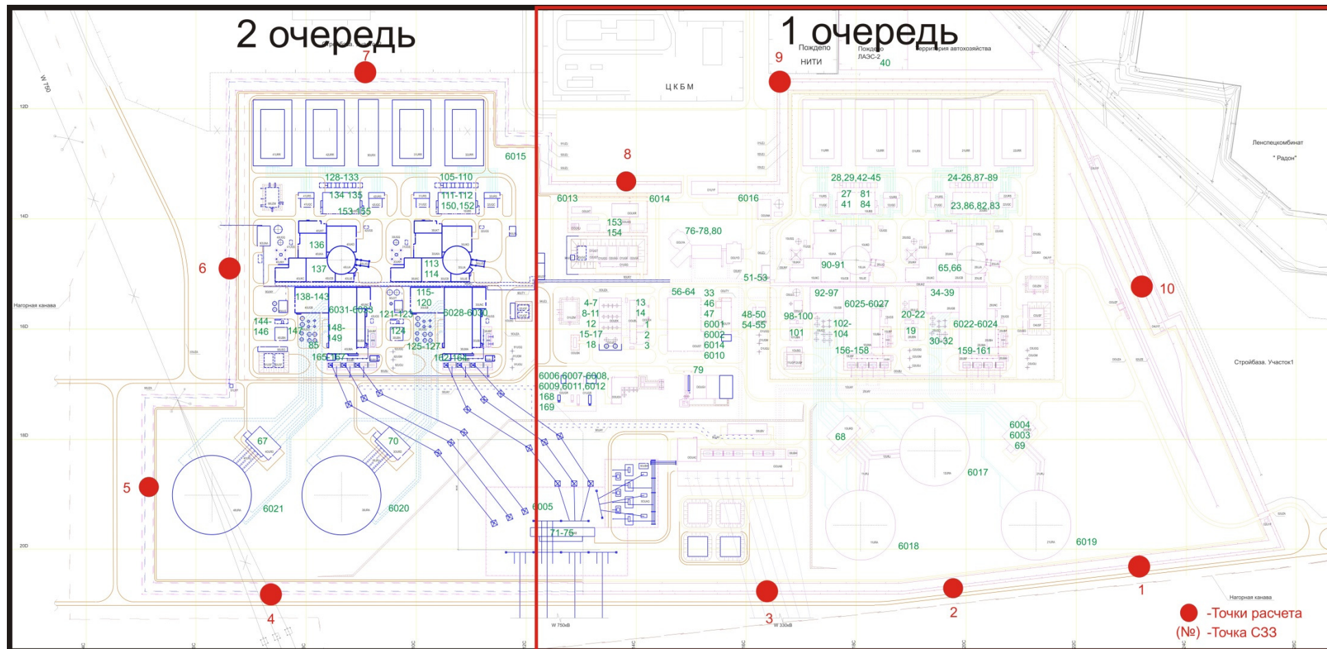
Рисунок 5.4.1.1.2 – Источники выбросов и расчетные точки рассеивания на площадке Ленинградской АЭС-2 (при эксплуатации)
