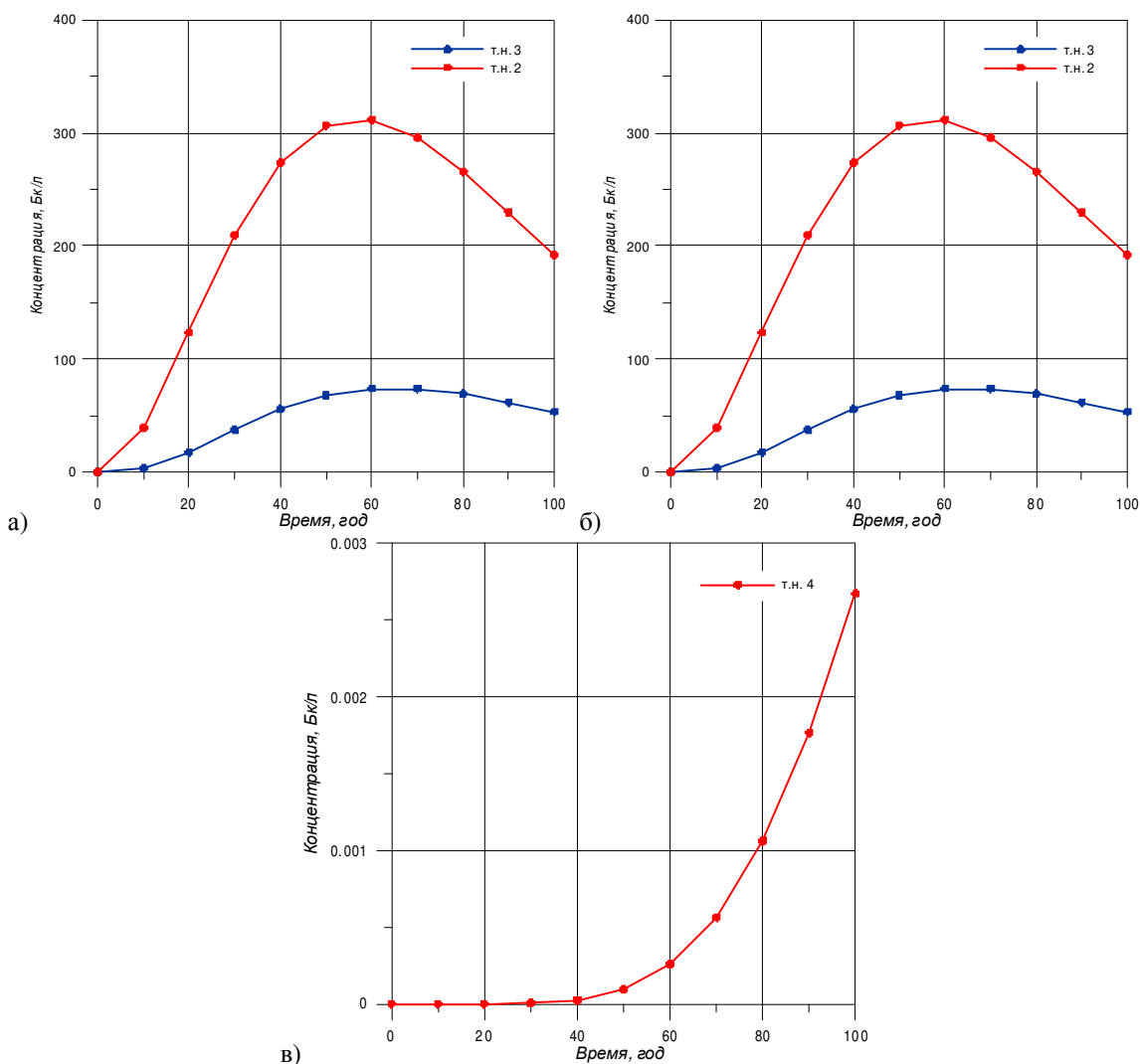
Рисунок 5.3.3.3.2 - Закономерности изменения концентрации Sr-90 при мгновенном попадании конденсата в водоносный горизонт (вариант 1).
