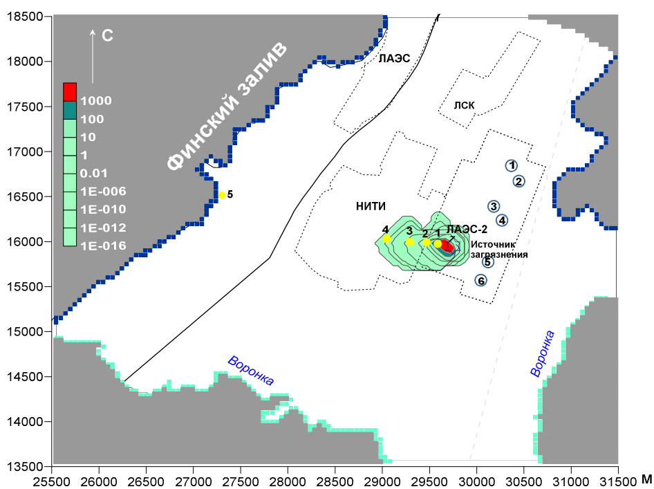
Рисунок 5.3.3.3.2 - Закономерности изменения концентрации Sr-90 при мгновенном попадании конденсата в водоносный горизонт (вариант 1).
