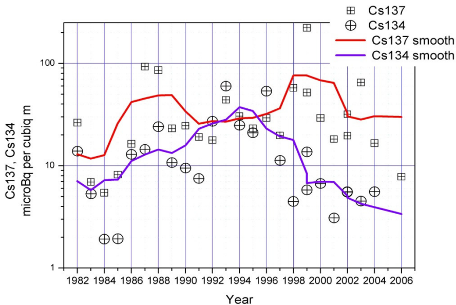
Рисунок 4.1.2.1.2.5 - Среднегодовая объемная активность 137 Cs и 134 Cs в воздухе на площадке ЛСК «РАДОН» (точка «1401»)
