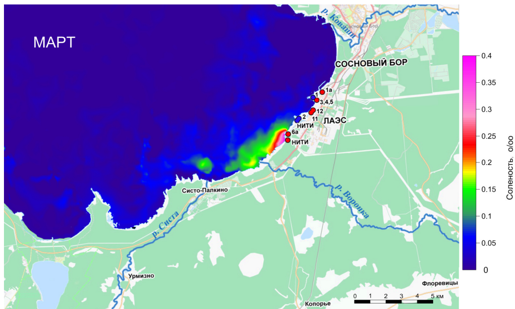
Рисунок 5.4.3.7 – Влияние сброса на распределение солености в Копорской губе (март): разница соленостей между сценариями 4 (сброс с ЛАЭС и ЛАЭС-2) и 2 (сброс только с действующей ЛАЭС)
