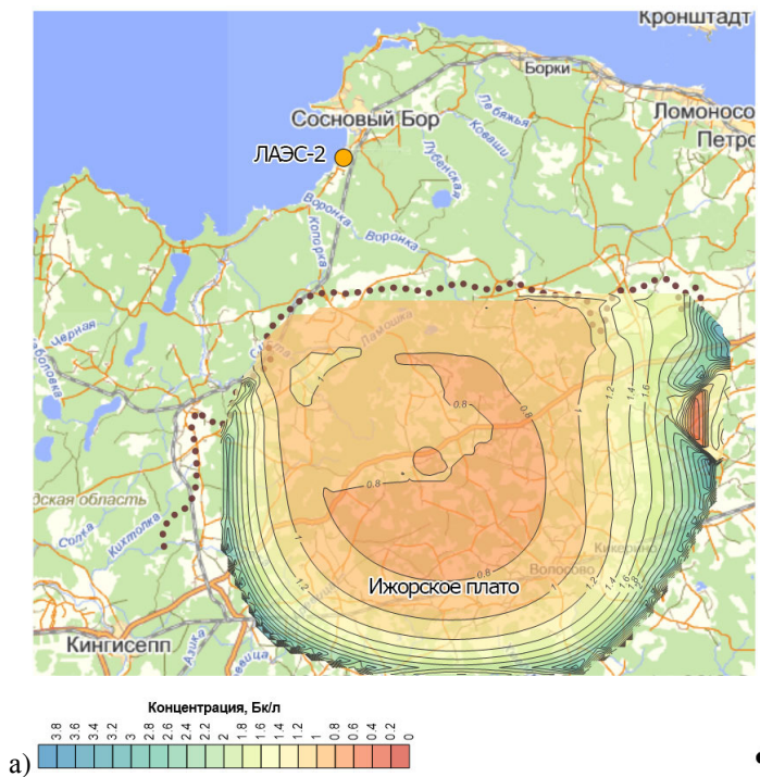
Рисунок 5.3.4.3.1 - Изменение концентрации радионуклидов в области разгрузки подземных вод по глинту Ижорского плато (консервативная оценка) а – Cs-137, б– Sr-90
