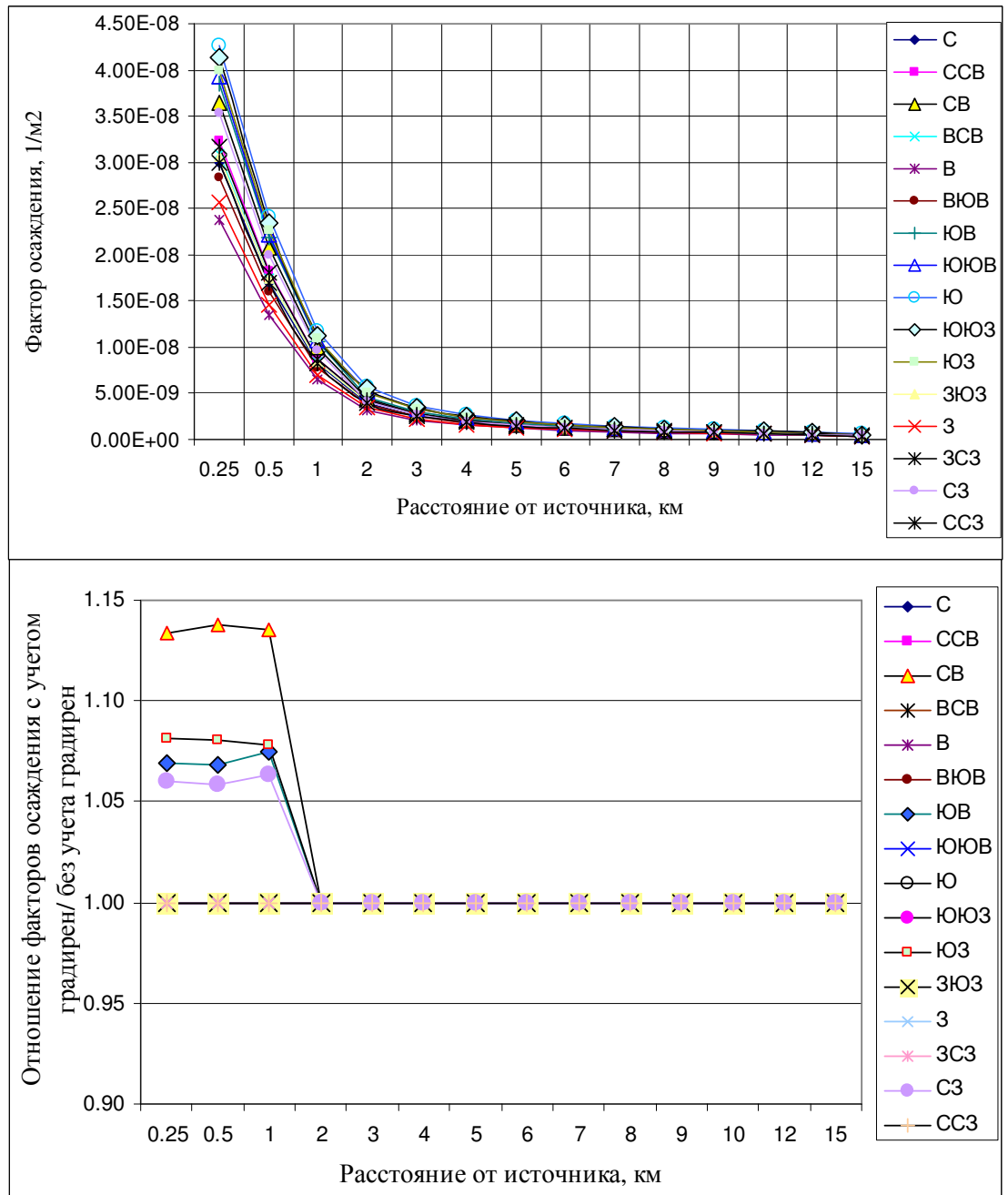
Рисунок 5.1.1.2.1.1 – Результаты расчета средних многолетних значений фактора осаднения ( 1/m^2 ) по 16 основным румбам ветра для источника в точке №1 (высота 33м) на турбинного острова второй очереди ЛАЭС-2 (блок 3) с учетом пароконденсатных факелов градирен (наверху) и относительный вклад этого эффекта (внизу).
