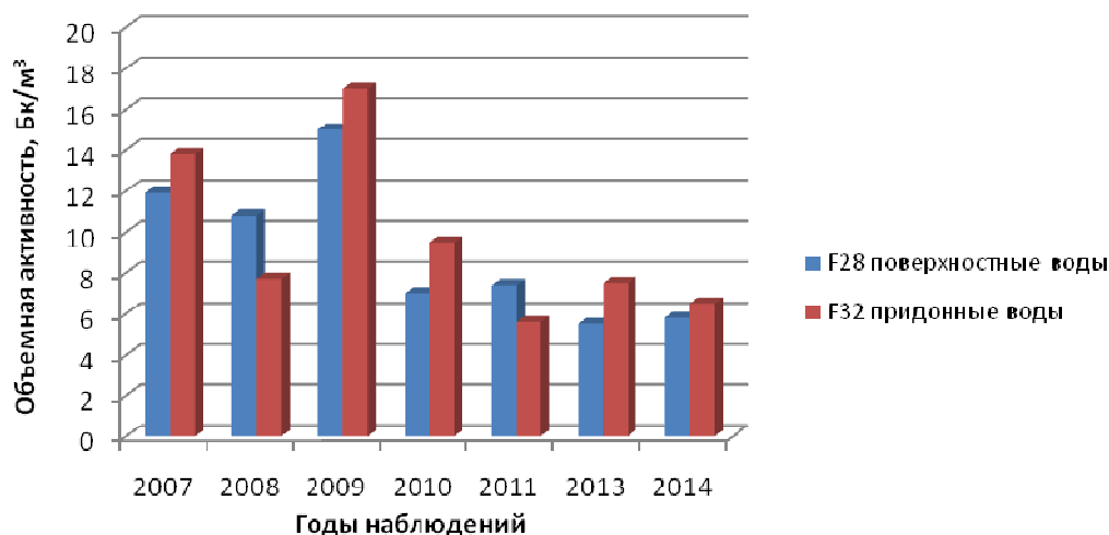
Рисунок 4.3.2.2.1.1.3 - Динамика концентрации ^{90}\text{Sr} в поверхностной и придонной воде Копорской губы ближней зоны размещения ЛАЭС-2 за период 2007 - 2014 г.
