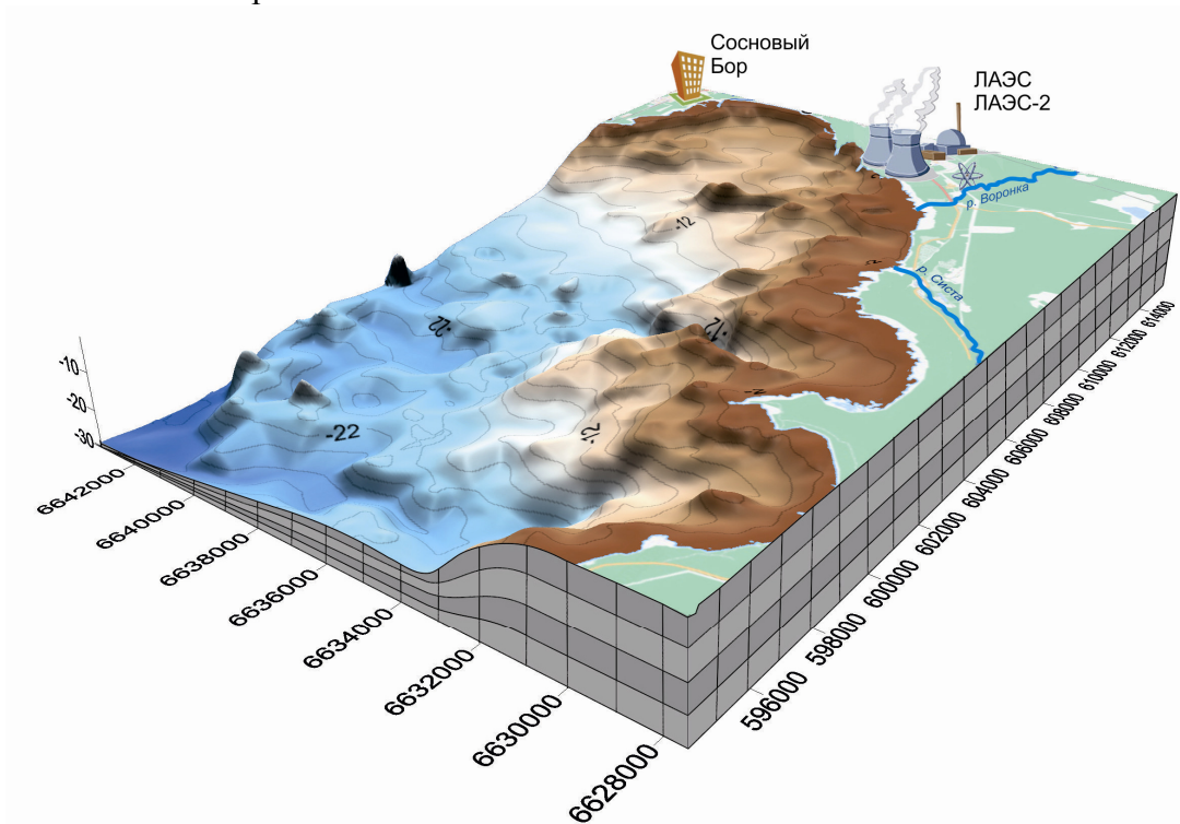
Рисунок 5.4.3.1 – Трехмерное представление модельной области
