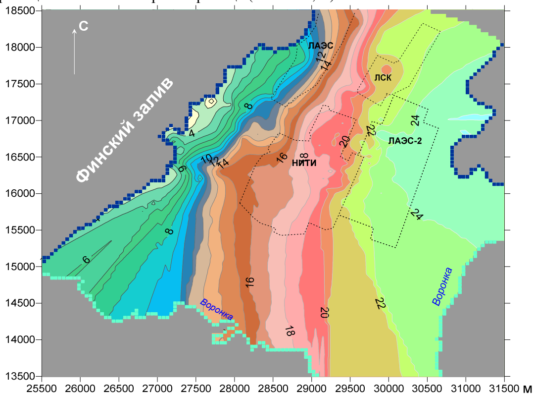
Рисунок 5.3.3.1.2.3.2 - Карта кровли четвертичных отложений (I-й расчетный слой)
