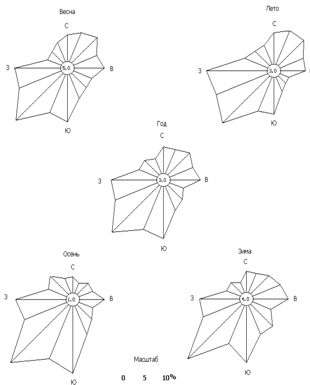
Рисунок 5.4.4.1.1 - Повторяемость направлений ветра по сезонам и за год по метеостанции Старое Гарколово
