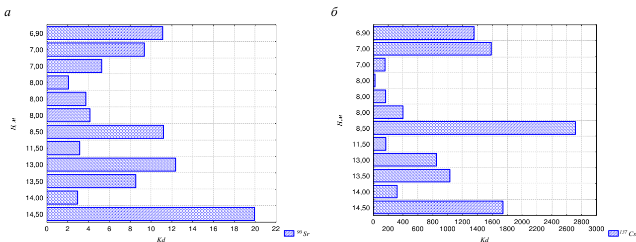
Рисунок 5.3.3.1.3.1.3 - Изменение коэффициента распределения с глубиной: а – 90 Sr, б – 137 Cs
