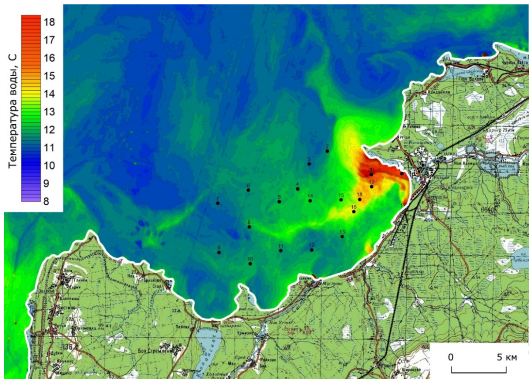
Рисунок 4.3.1.2.1.5 – Распределение тепловых ореолов на поверхности Копорской губы (13:00, 24.05.2014 г.)
