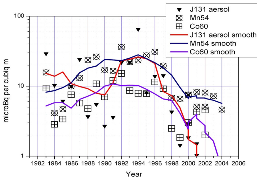
Рисунок 4.1.2.1.2.3 - Среднегодовая объемная активность ^{131}\text{I} (аэрозоль) ^{60}\text{Co} и ^{54}\text{Mn} в воздухе на промплощадке АЭС (точка «100»)
