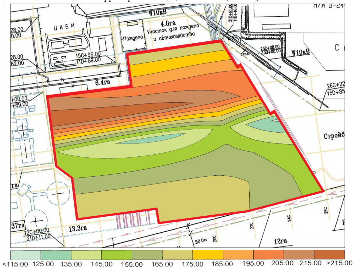
Рисунок 4.2.2.5.3 - Удельная активность радионуклидов на территории площадки ЛАЭС-2 (Бк/кг)
