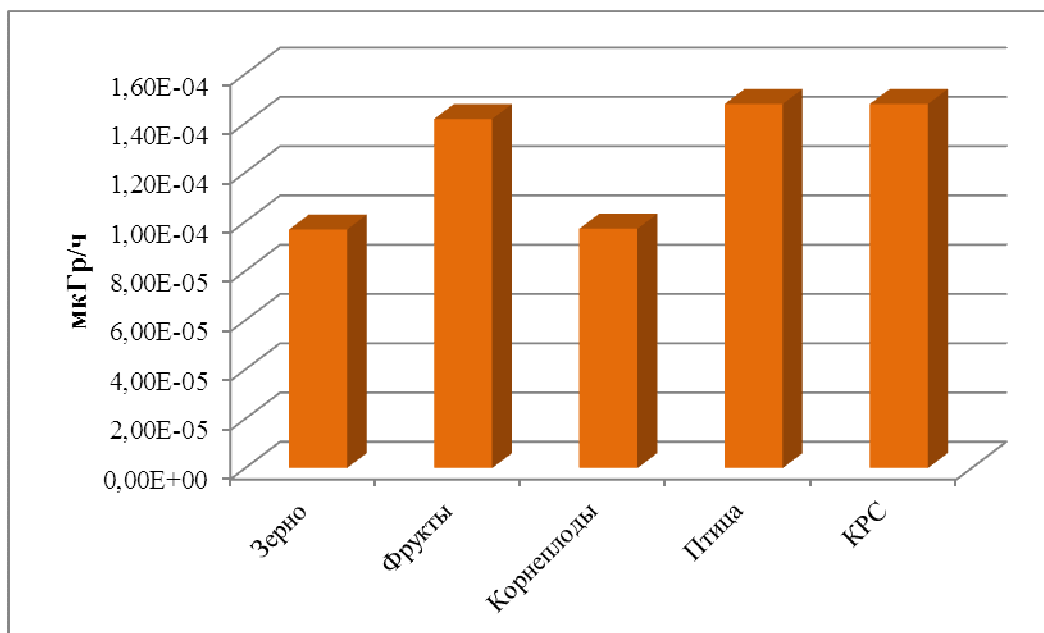
Рисунок 5.1.1.5.1 - Суммарные дозовые нагрузки на компоненты агроэкосистем
