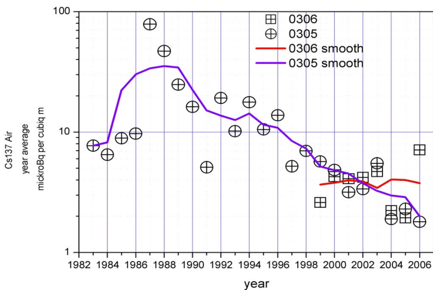
Рисунок 4.1.2.1.2.6 - Среднегодовая объемная активность 137 Cs в воздухе на территории г. Сосновый Бор (точки «0305» и «0306»)
