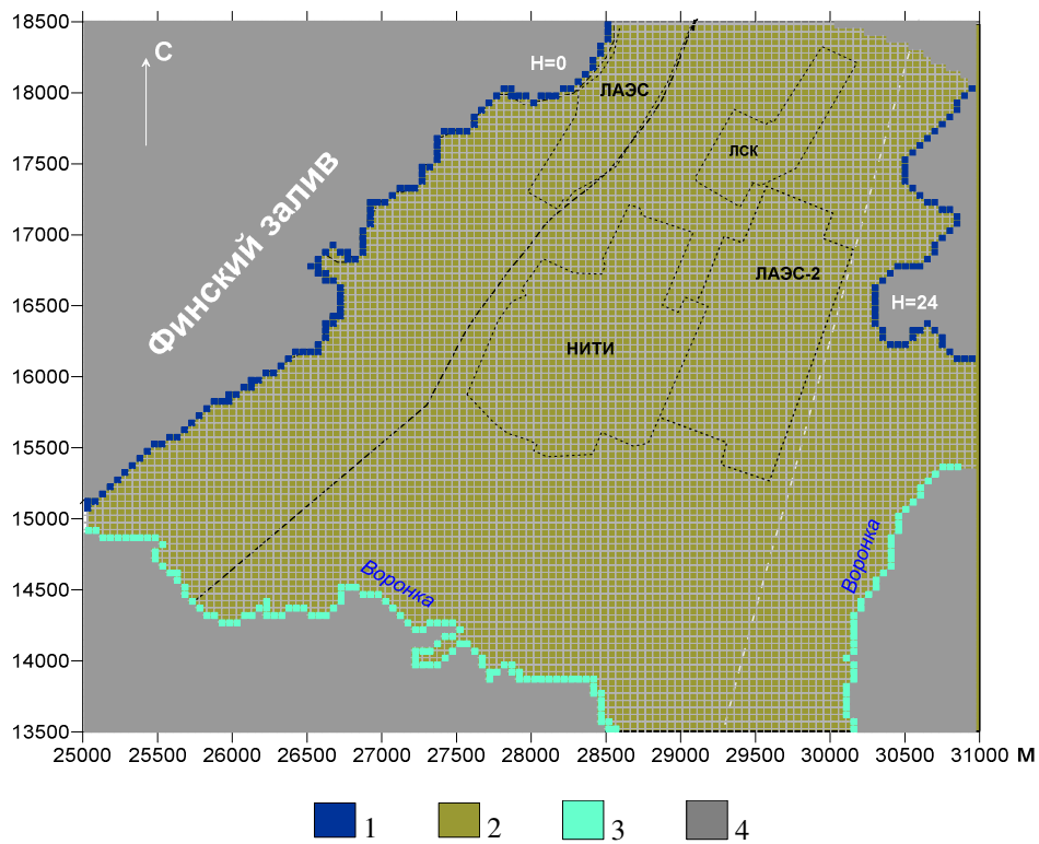
Рисунок 5.3.3.1.2.3.1 - Схема задания граничных условий
