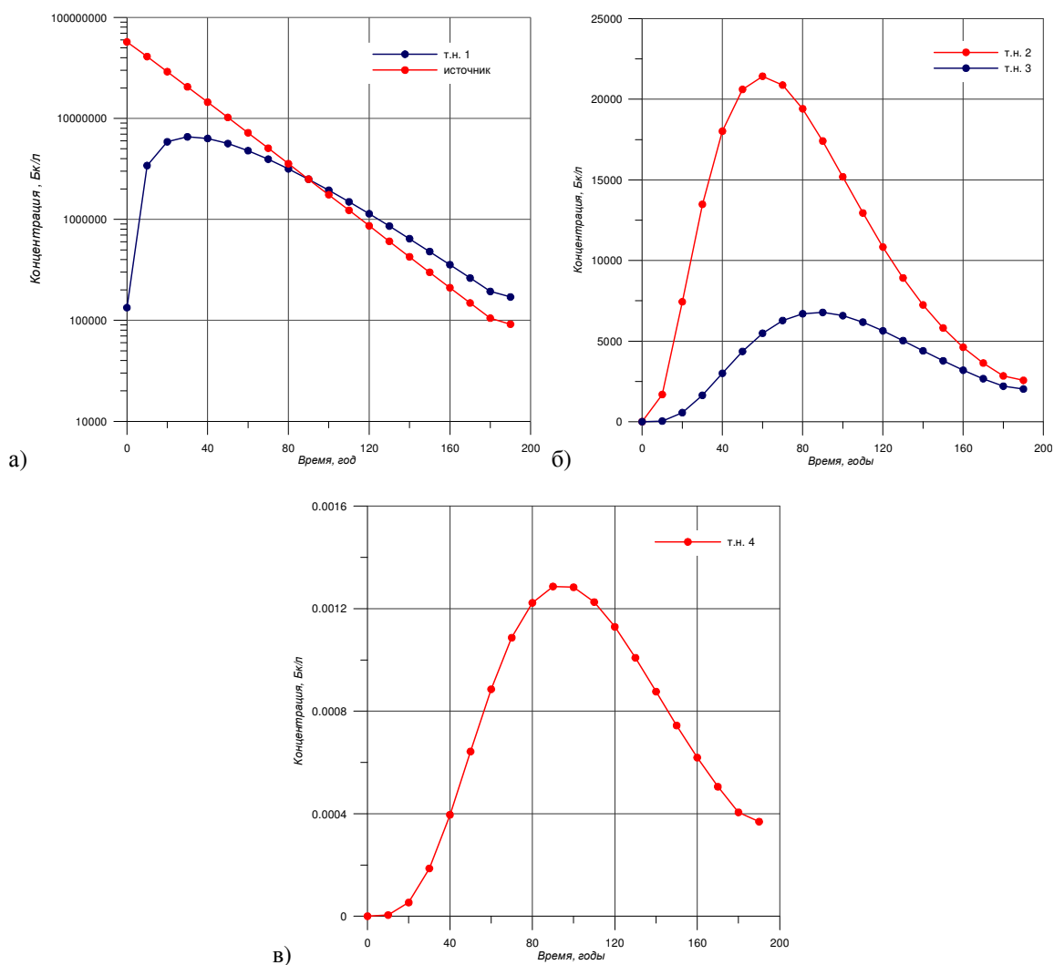
Рисунок 5.3.3.3.5 - Закономерности изменения концентрации Sr-90 при мгновенном попадании конденсата в водоносный горизонт (варианты 2 и 3).
