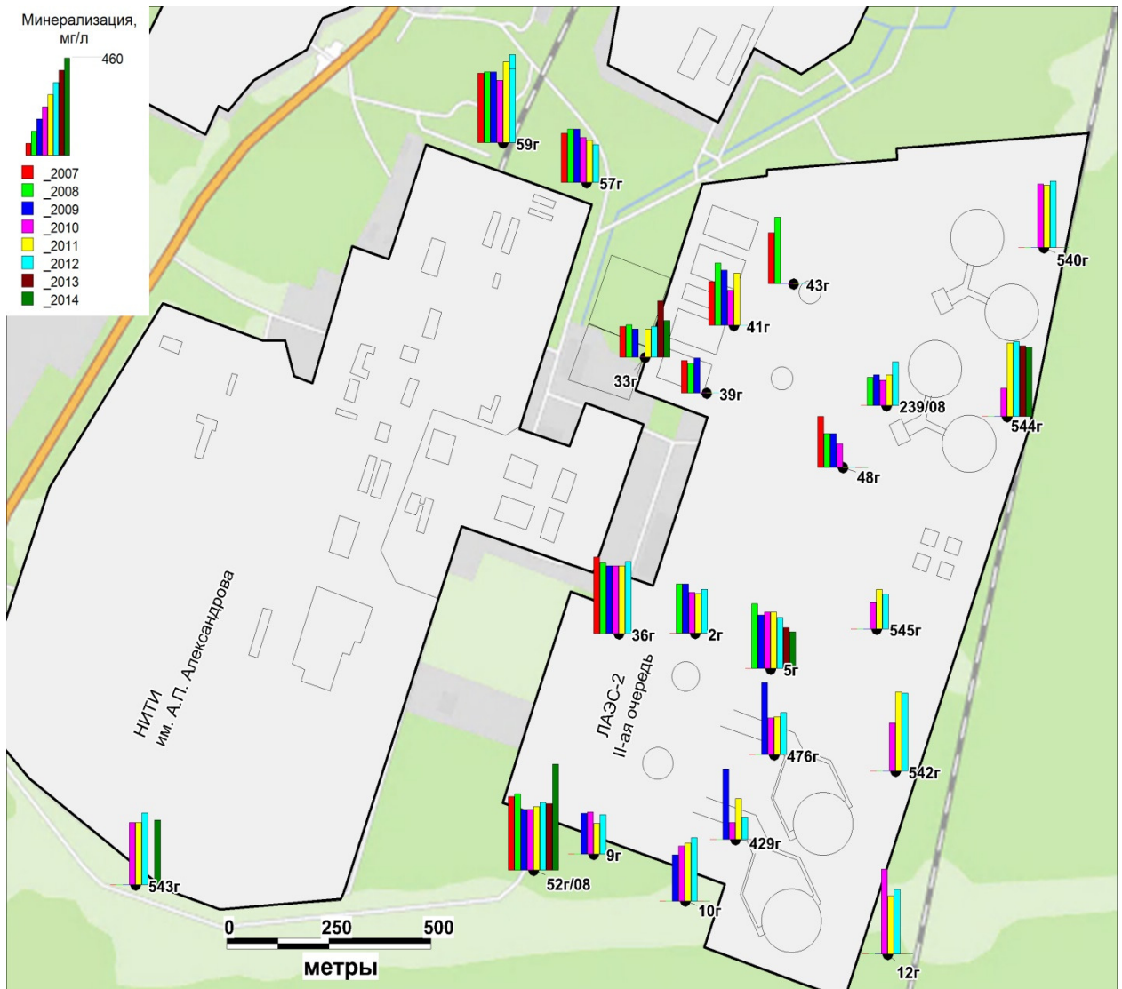
Рисунок 4.3.1.2.7.1.2 – Изменение среднегодовых значений минерализации подземных вод верхней и средней зон ломоносовского горизонта
