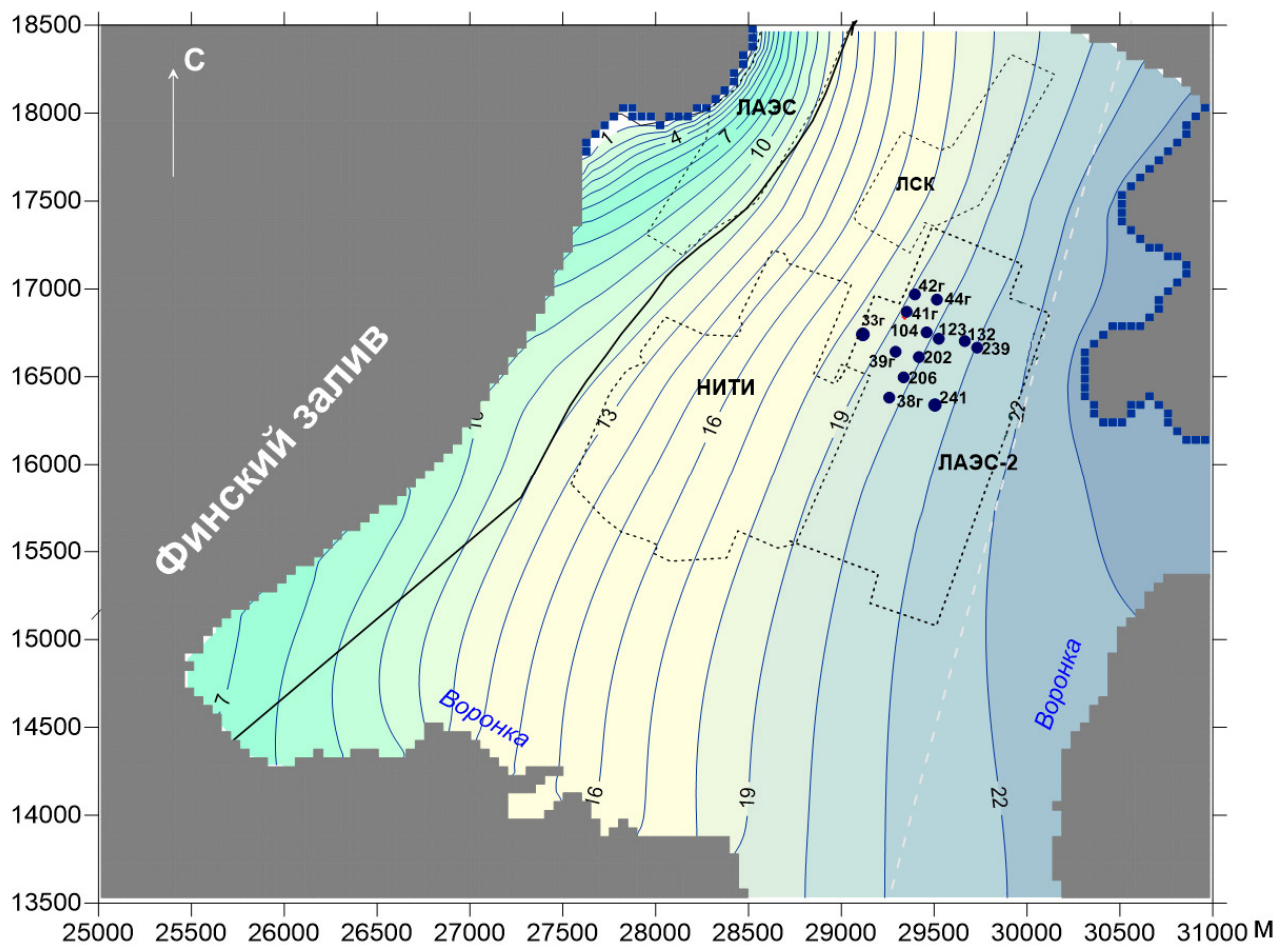
Рисунок 5.2.3.1.2.5.1 - Модельное распределение напоров в ломоносовском водоносном горизонте
