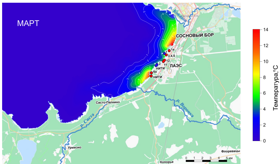
Рисунок 5.4.3.4 – Среднее месячное распределение температуры в марте на поверхности Копорской губы в «фоновом» сценарии 1 (верхний фрагмент), сценарии 2 (современное состояние ЛАЭС) (средний фрагмент) и вклад ЛАЭС (разница температур между сценариями 2 и 1) в естественный режим (нижний фрагмент)
