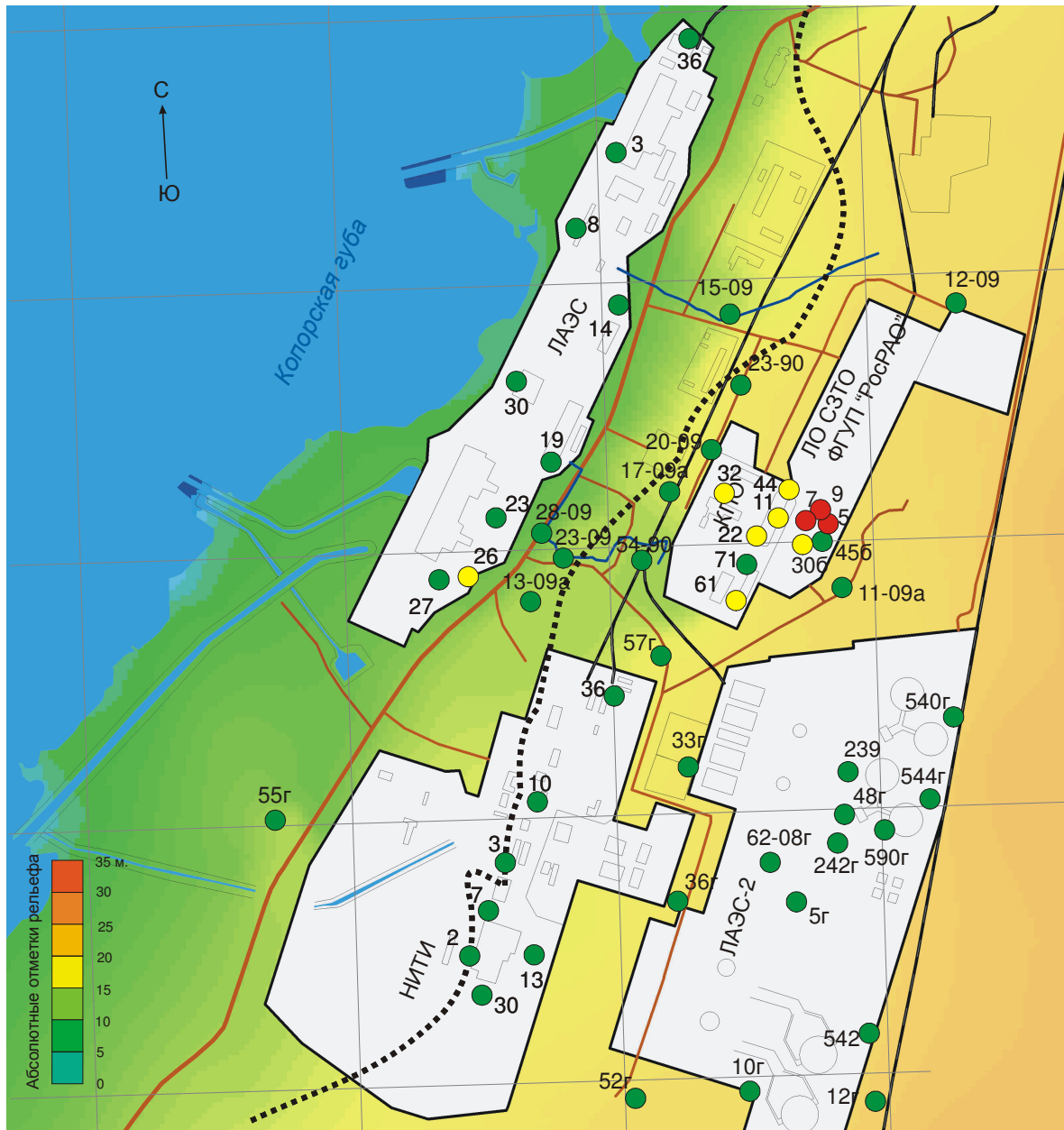
МАСШТАБ 0 200 400 600 800 1000 м. 52г 26 7 ● 1 ● 2 ● 3 - - - 4 Примечание—1–3 – скважины с объемной активностью ^{90}\text{Sr} и ^{137}\text{Cs} : 1 – менее 0,1 Бк/л (близкой к фоновой); 2 – более 0,1 Бк/л (надфоновой); 3 – выше УВ по НРБ--99/2009; 4 – линия выклинивания нижнекембрийского горизонта.
