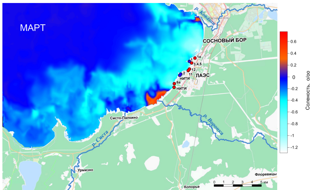
Рисунок 5.4.3.5 – Влияние сброса на распределение солености в Копорской губе (март): разница соленостей между сценариями 2 и 1
