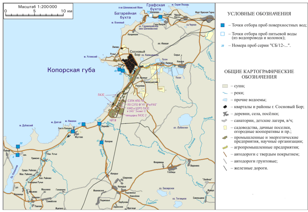
Рисунок 4.3.2.2.1.1.5 - Схема отбора проб поверхностных и питьевых вод для определения объемной активности ^{90}\text{Sr} в ЗН ЛАЭС-2 за 2012 г.
